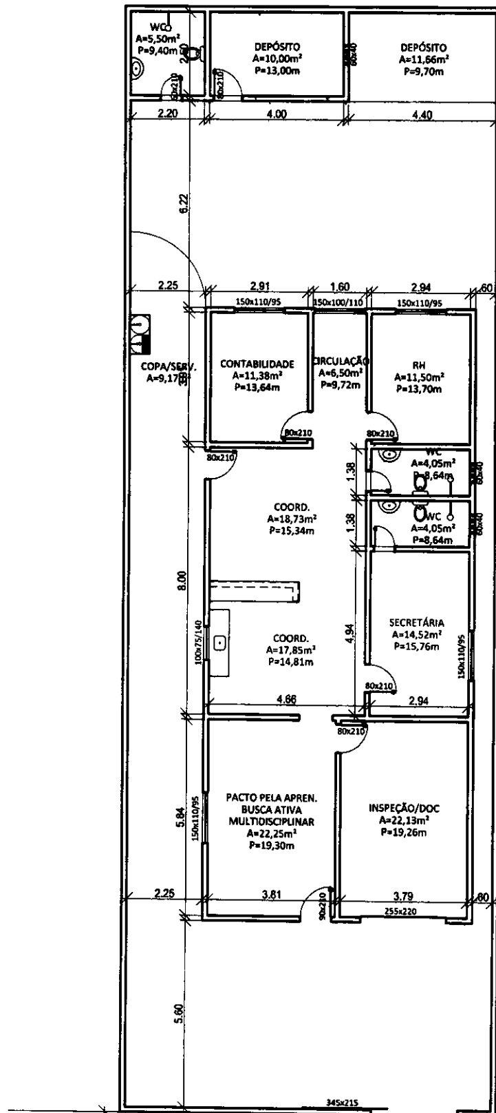
PLANTA BAIXA ESCALA 1-150
